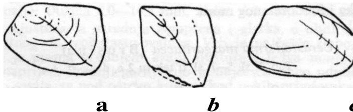
SI. (Text fig.) 1. Shematski crtež vrsta Congeria vugroveci n. sp. (a), C. banatica (b) i Cerastoderma protracta (c) — za usporedbu.
