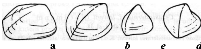
SI. (Text-fig.) 2. Varijabilnost oblika vrsta Cerastoderma protracta (a, b) i C. margaritacea (c, d).
